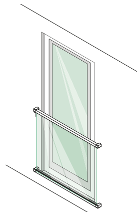
Montaje en la fachada con tubo angular horizontal
